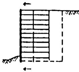
(d) Keruntuhan Geser
