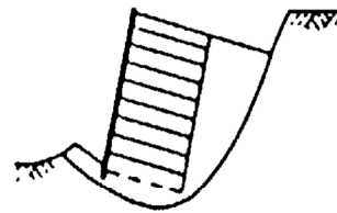
(f) Longsor Menyeluruh
